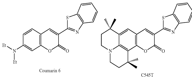
C545T
